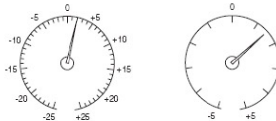
Figura 14 La escala de la izquierda es inadecuada cuando se quieren medir valores entre -5 y 5
