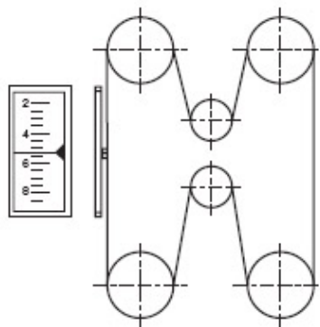
Figura 6 Escala vertical de índice fijo
