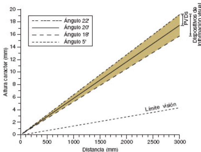
Figura 8 Valores de ángulo de visión recomendados por la UNE-EN 894-2 y la UNE-EN 29241-3 para dispositivos de información visual y pantallas de visualización respectivamente
